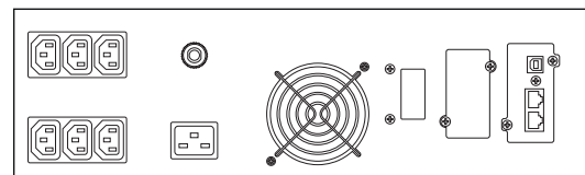
Задняя панель ИБП в стойку ЮНИОР ПРО РТ 2000 и 3000 ВА 3U
